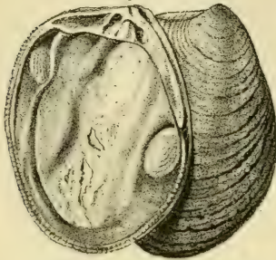
Fig. 151. — Crassinella obliquata , .
